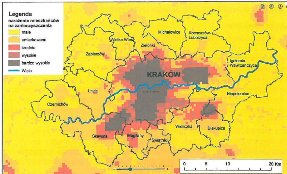
Rysunek 19. Narażenie mieszkańców na zanieczyszczenia powietrza
