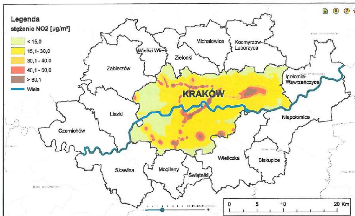
Rysunek 21. Stężenie średnioroczne dwutlenku azotu (NO 2 ) [µg/m 3 ]
